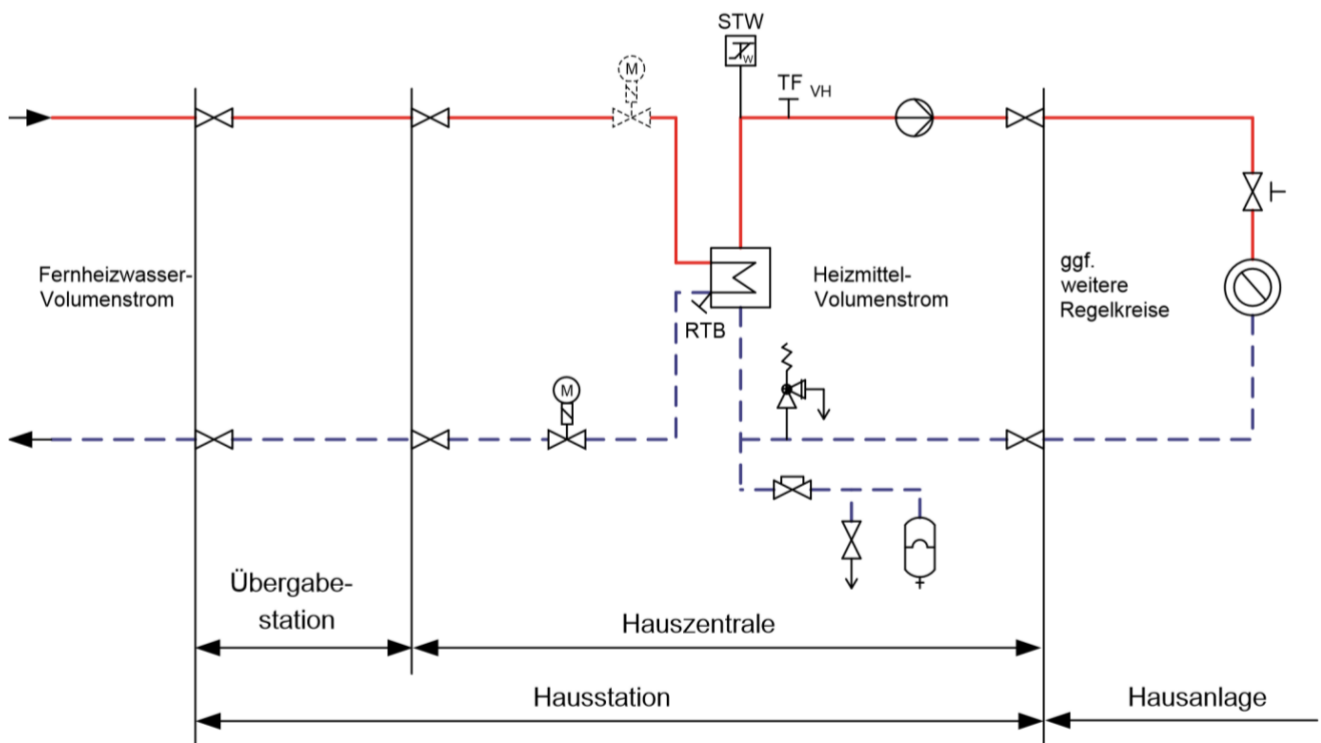
Abbildung 12: Hauszentrale-Raumheizung Prinzipialschaltbild für den indirekten Anschluss
